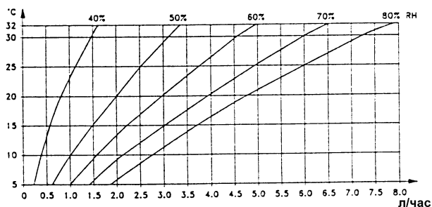
Рис.47 График зависимости производительности осушения CDS 6000 от температуры и влажности воздуха
