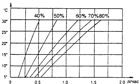
Рис.23 График зависимости производительности осушения CD 1800 от температуры и влажности воздуха
