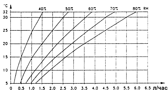
Рис.46 График зависимости производительности осушения CDS 3000 от температуры и влажности воздуха
