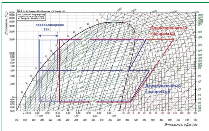
Рис. 1. Пример диаграммы цикла холодильной установки с двухступенчатым поршневым компрессором (в сравнении с циклом установки с одноступенчатым компрессором)
