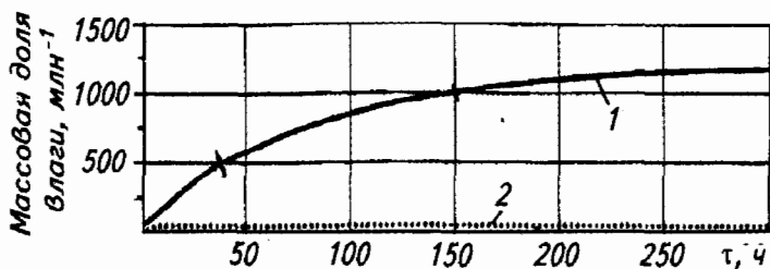
Рис. 11. Поглощение влаги полиэфирным маслом (1) по сравнению с минеральным (2) в частях на миллион по массе при температуре 25 °C и относительной влажности 50 % (по данным фирмы «Copeland»)
