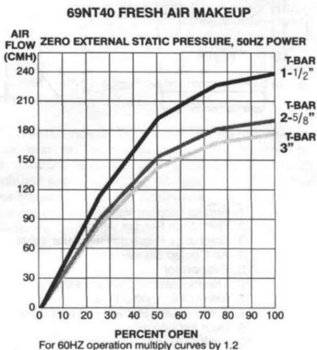
Рис.: Подача свежего воздуха в контейнер, агрегат 69ЭТ40. Ось Y - поток воздуха, ось X - процент открытия крышки. Данные для нулевого внешнего давления и питания 50Гц. Для 60Гц, умножить значения кривых на 1,2.
