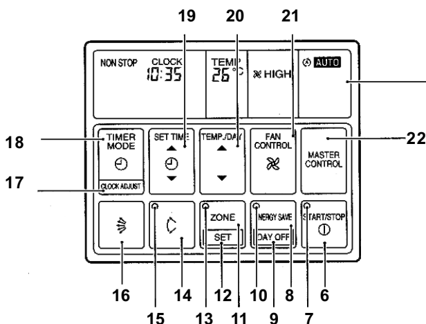
Рис.5 Дисплей
