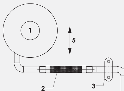
РИС.1 СИСТЕМА С ОДНИМ ВИБРОИЗОЛЯТОРОМ
