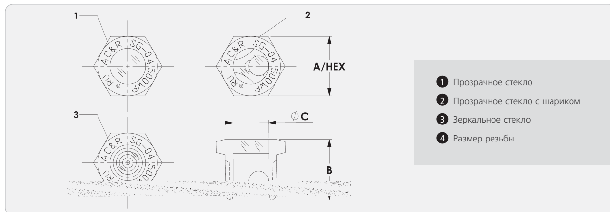
СТЕКЛЯННЫЕ УРОВНЕМЕРЫ
