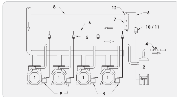
СИСТЕМА РЕГУЛИРОВАНИЯ ПОДАЧИ МАСЛА НИЗКОГО ДАВЛЕНИЯ
