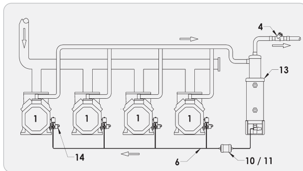
СИСТЕМА РЕГУЛИРОВАНИЯ ПОДАЧИ МАСЛА ВЫСОКОГО ДАВЛЕНИЯ
