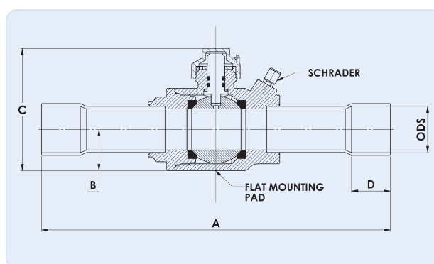
ШАРОВЫЙ КЛАПАН СЕРИИ 907
