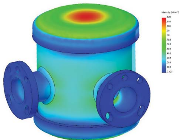
FEA – РЕГУЛЯТОР УРОВНЯ МАСЛА
