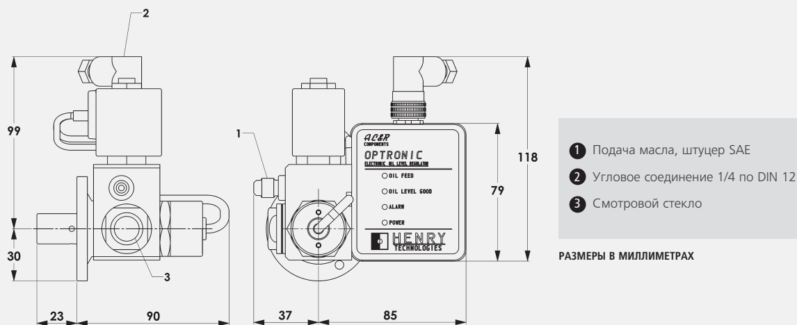
ОПТОЭЛЕКТРОННЫЙ РЕГУЛЯТОР УРОВНЯ МАСЛА
