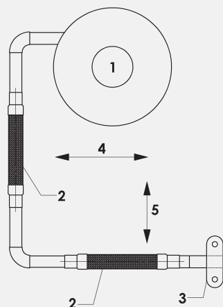
РИС.2 СИСТЕМА С ДВУМЯ ВИБРОИЗОЛЯТОРОМ
