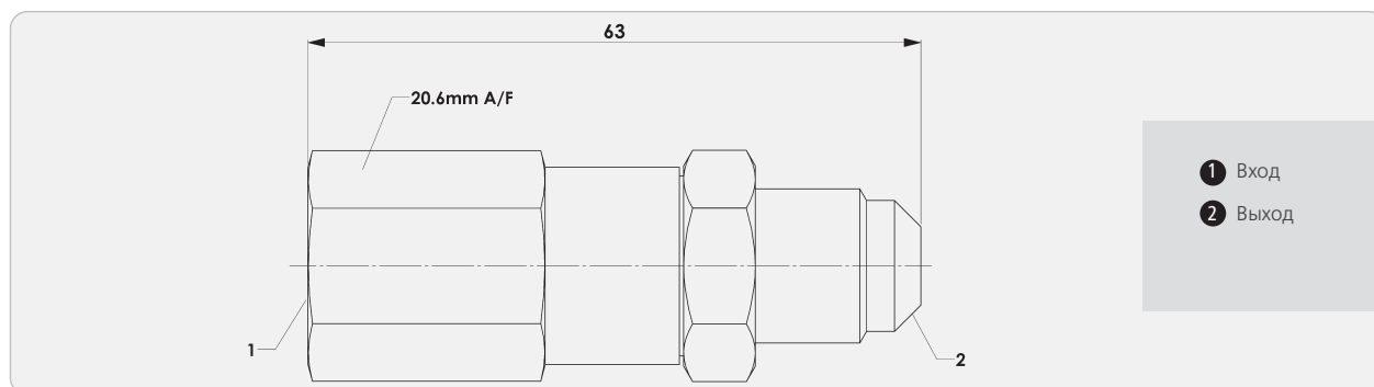
ДИФФЕРЕНЦИАЛЬНЫЙ КЛАПАН
