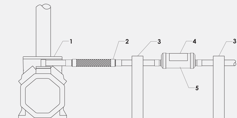
ПРАВИЛЬНОЕ КРЕПЛЕНИЕ ШУМОПОГЛОЩАЮЩЕГО УСТРОЙСТВА
