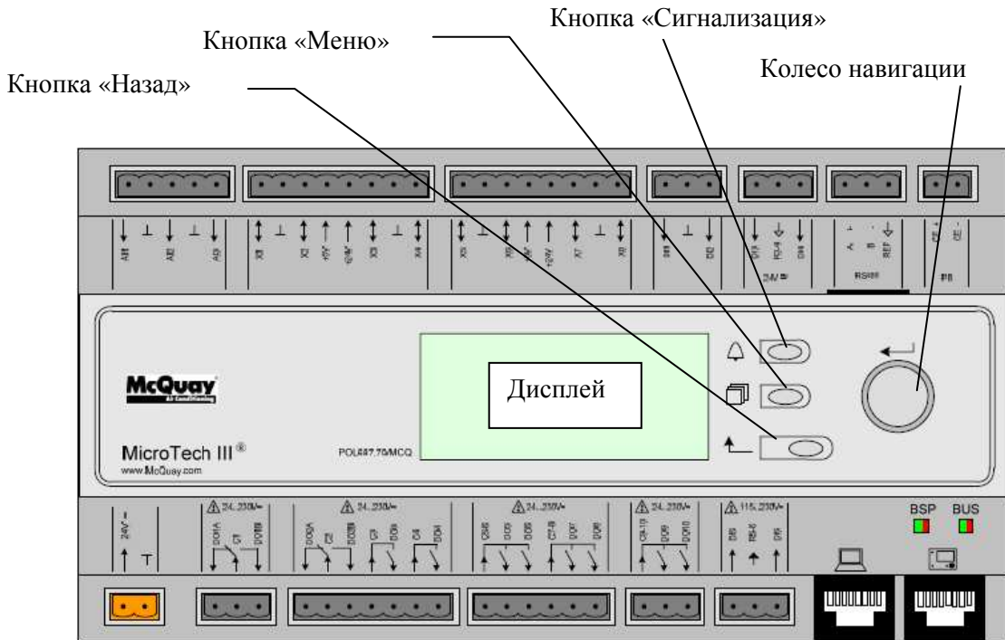
Рис. 7. Контроллер агрегата
