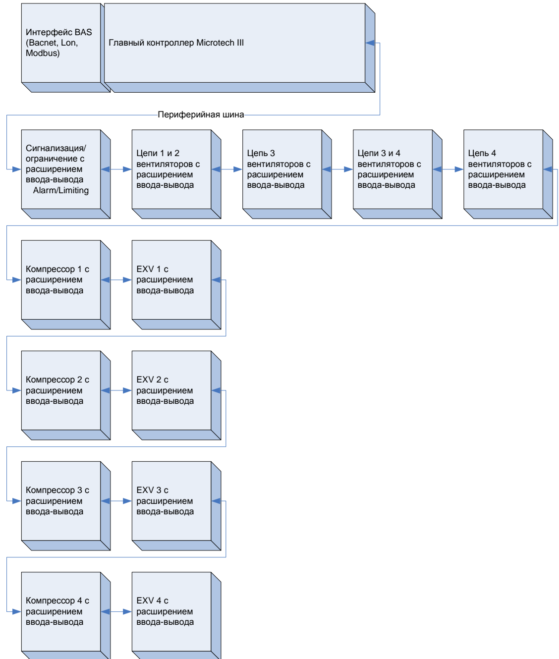
Рис. 4. Архитектура системы
