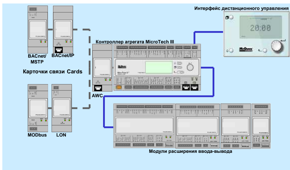
Рис. 6. Аппаратная структура
