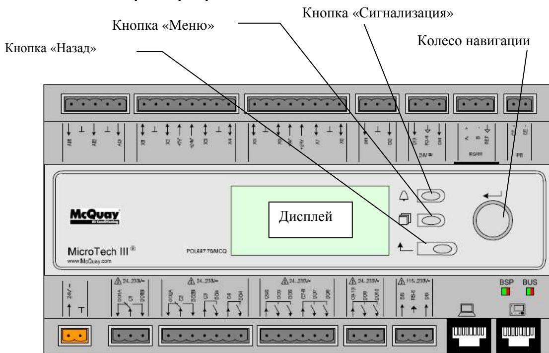
Рис. 6. Контроллер агрегата
