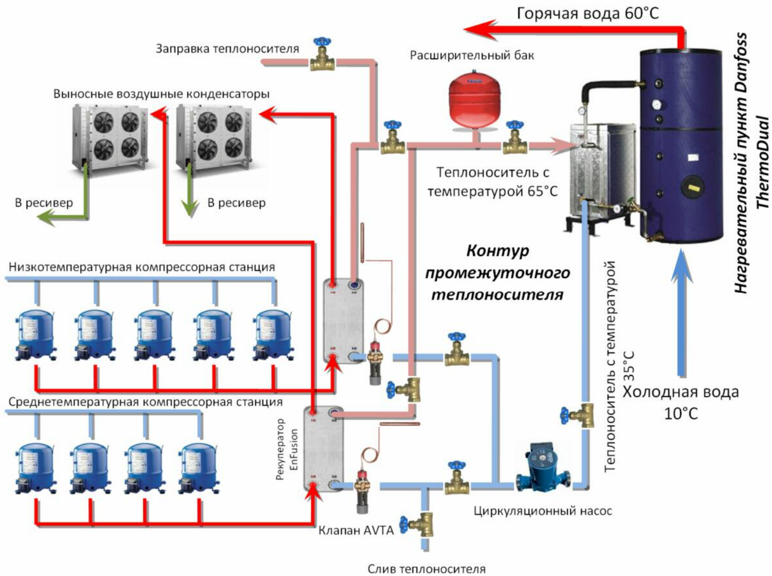
Принципиальная схема системы рекуперации Danfoss.
