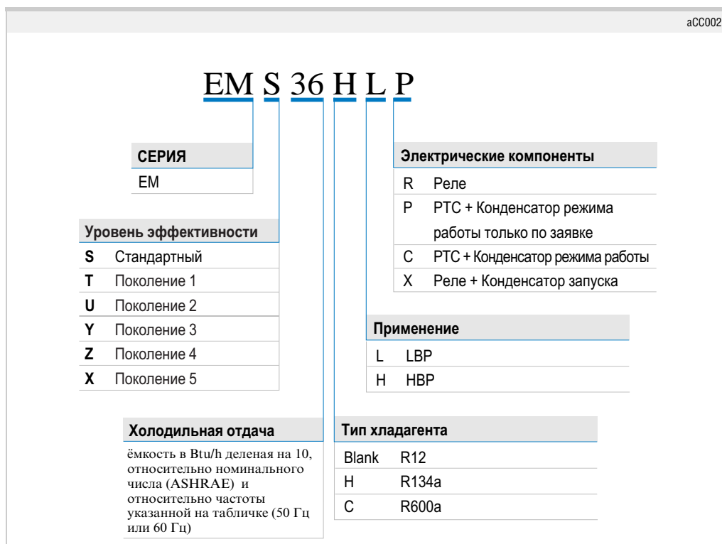
рис. 6b Типовой Код Компрессора серии EM
