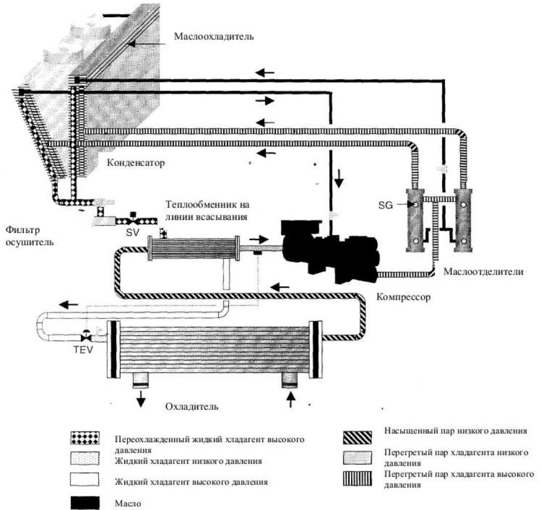
Рисунок 2.1 Пневмогидравлическая схема хладагента
