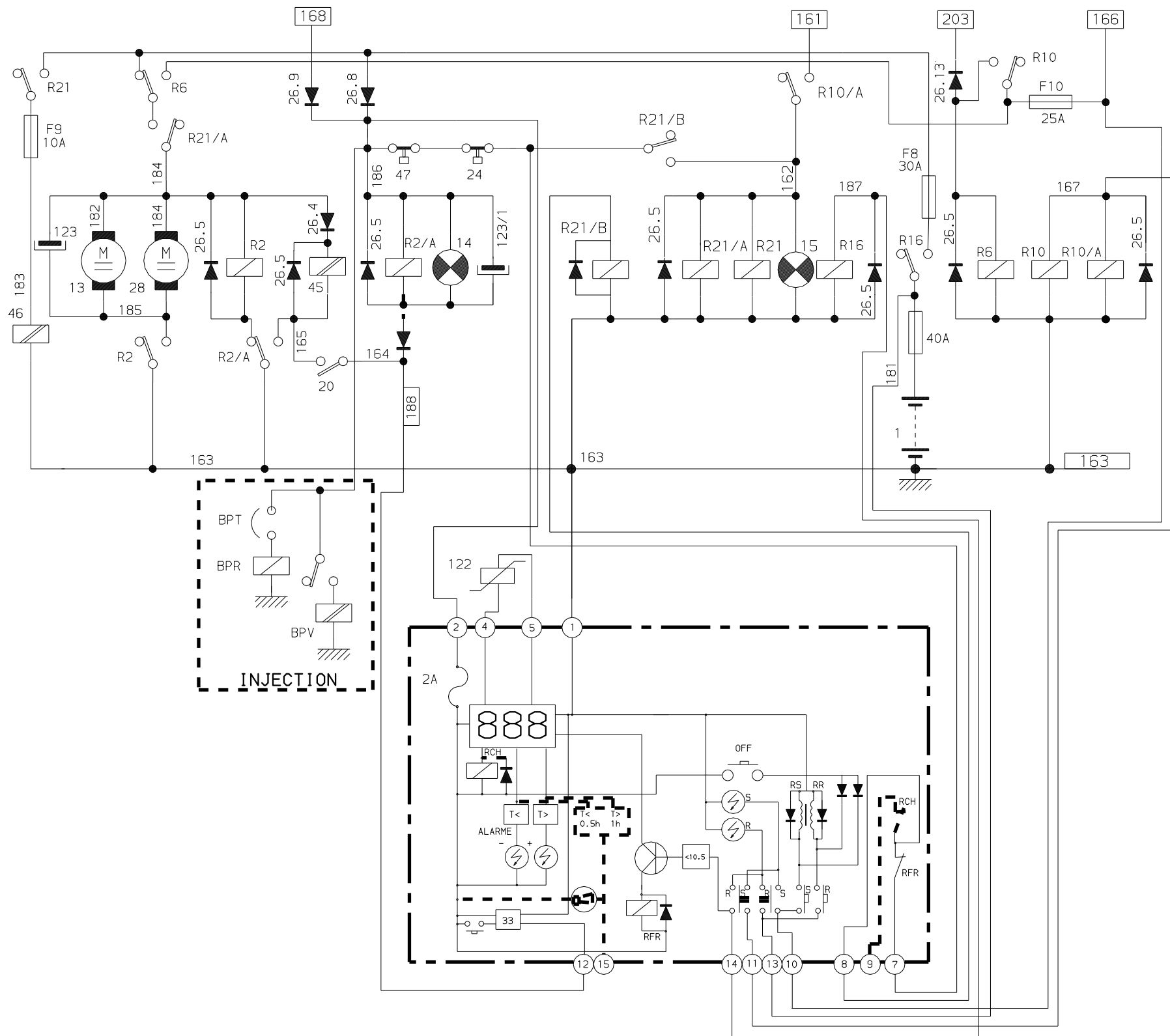
SCHEMA ELECTRIQUE DE PRINCIPE
