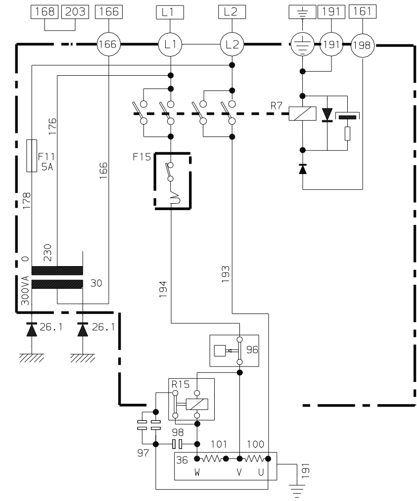
ESQUEMA ELECTRIICO DE PRINCIPIO
