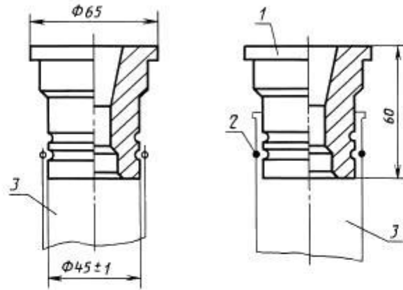
1 — патрубок; 2 — резиновое зажимное кольцо; 3 — презерватив
