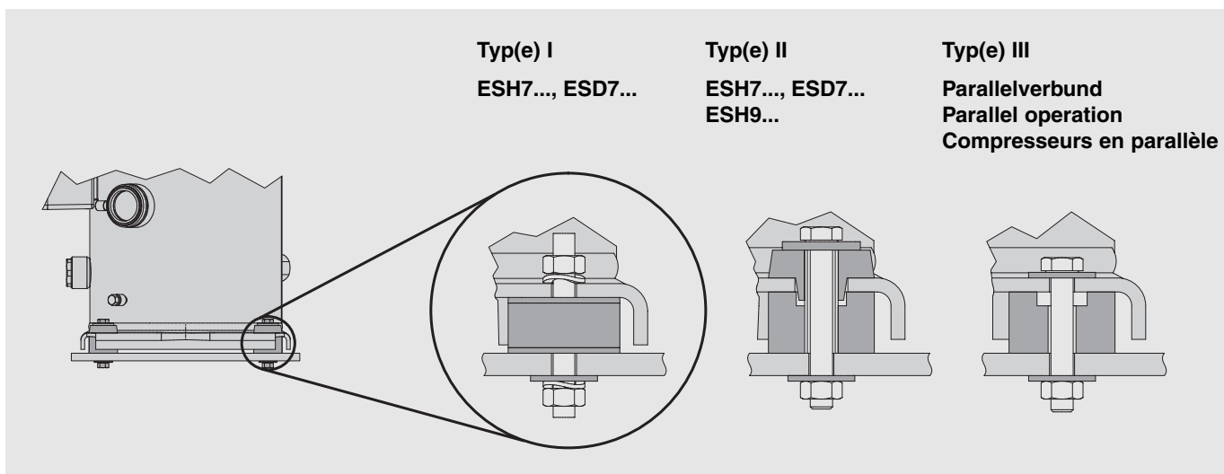
Abb. 2 Schwingungsdämpfer
