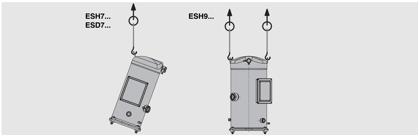
Abb. 1 Verdichter anheben
