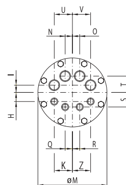
TBE../4 4 контура - CIRCUITS
