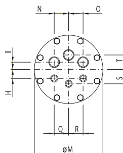
TBE../3 3 контура - CIRCUITS
