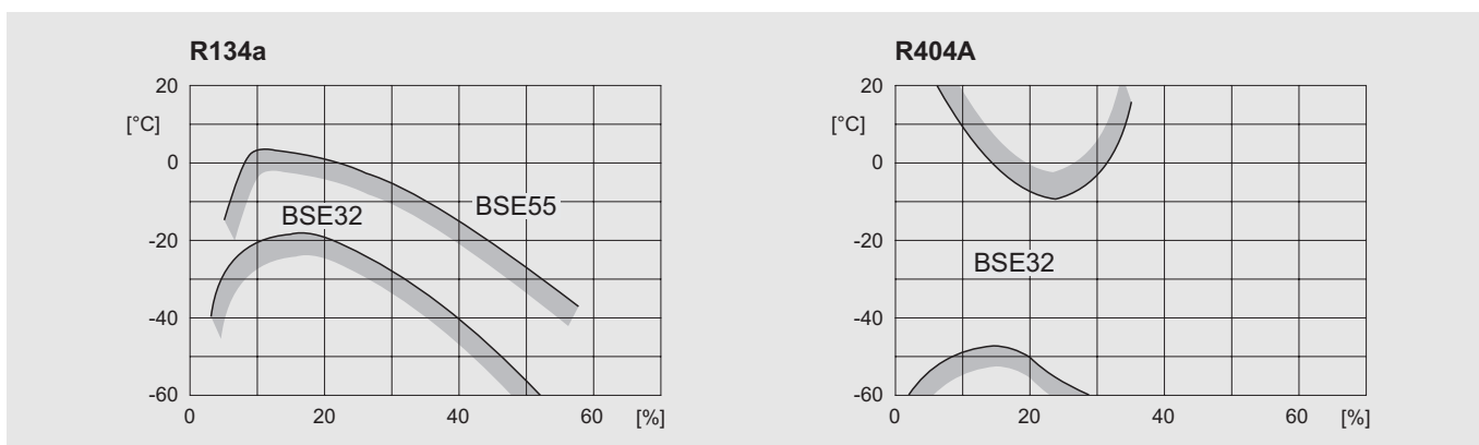
Abb. 1 Mischungsgrenzen Gewichtsanteil Öl im Kältemittel
