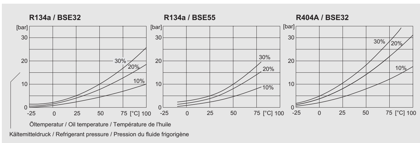
Abb. 2 Kältemittel-Konzentration im Öl in Abhängigkeit von Kältemitteldruck und Öltemperatur
